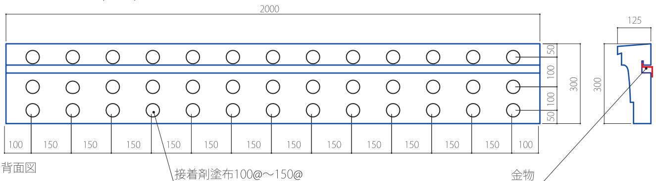
接着剤の位置例(図1)
